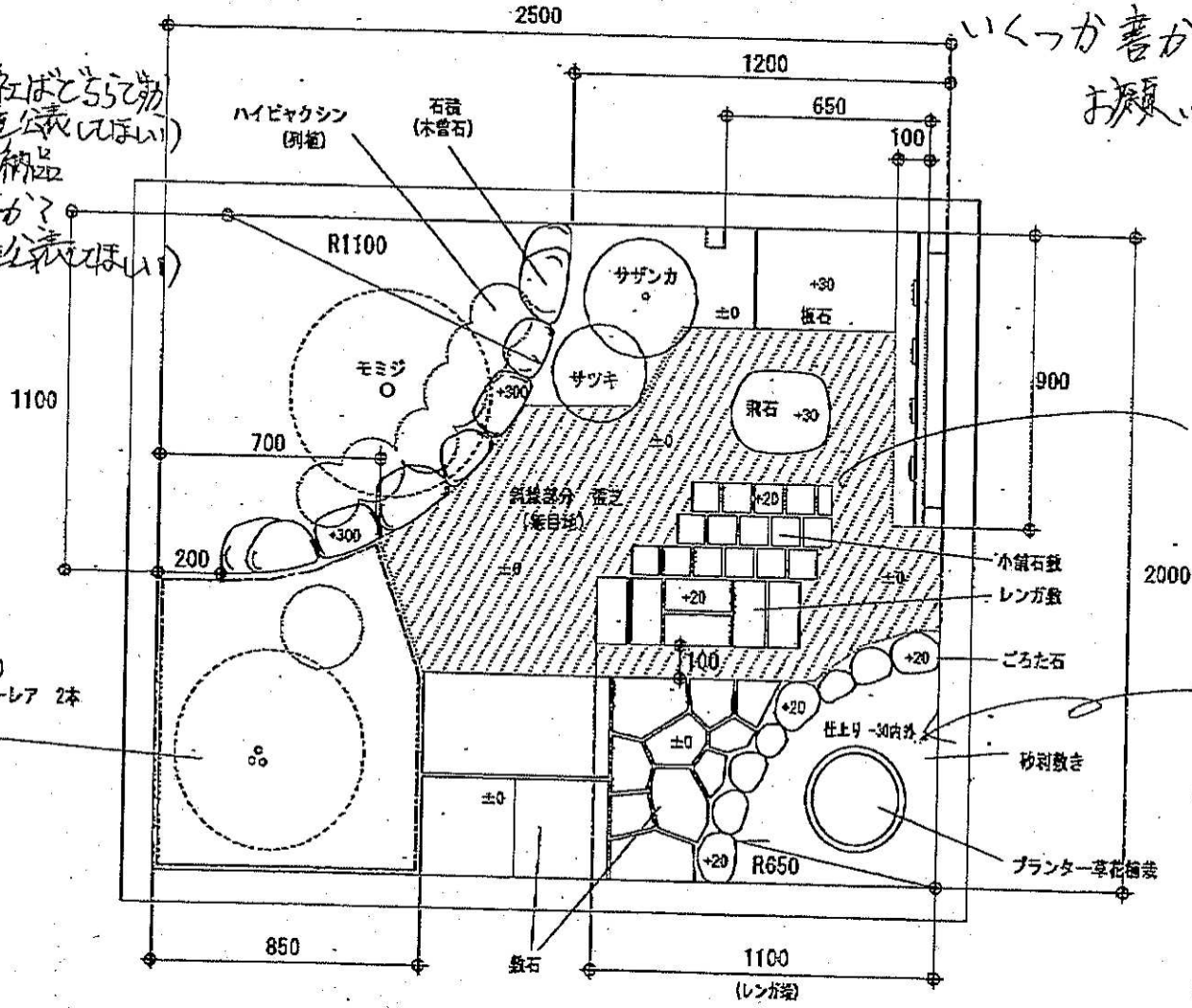
平面図 1:20
